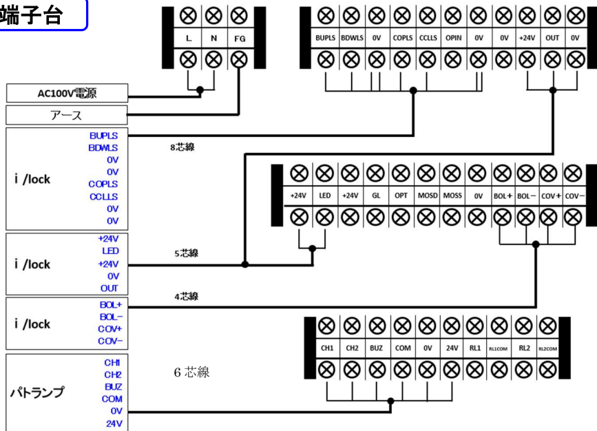
端子台
